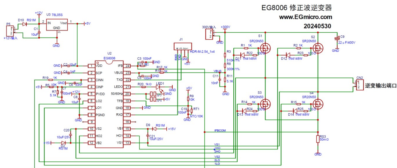
图 6-1. EG8006 典型应用原理图
