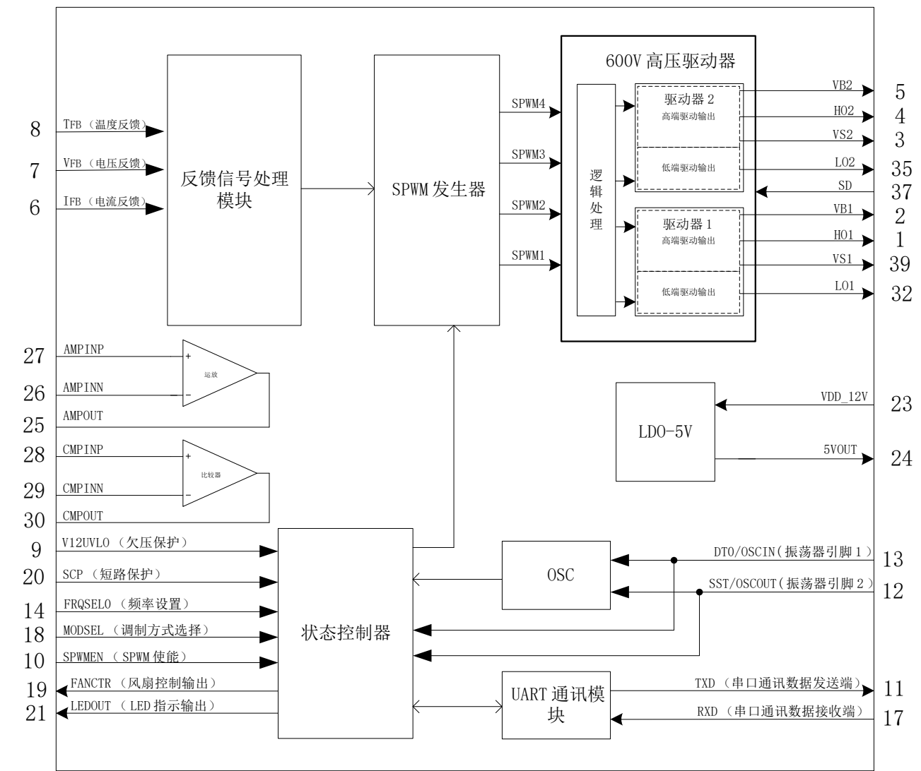
图 5-1. EG8015 结构框图
