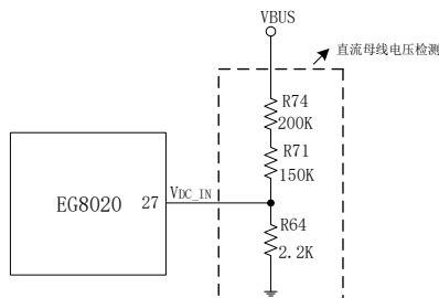
图 8.5a EG8020 的直流母线电压检测电路
