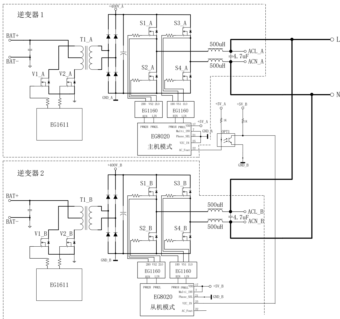
图 10-a.单相逆变器并机示意图
