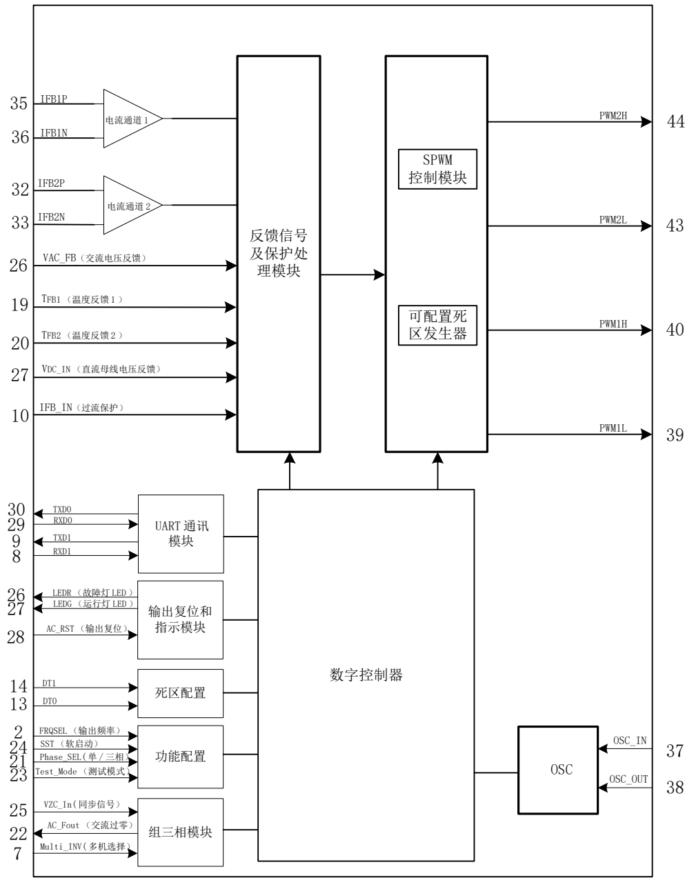
图 5-1. EG8020 结构框图
