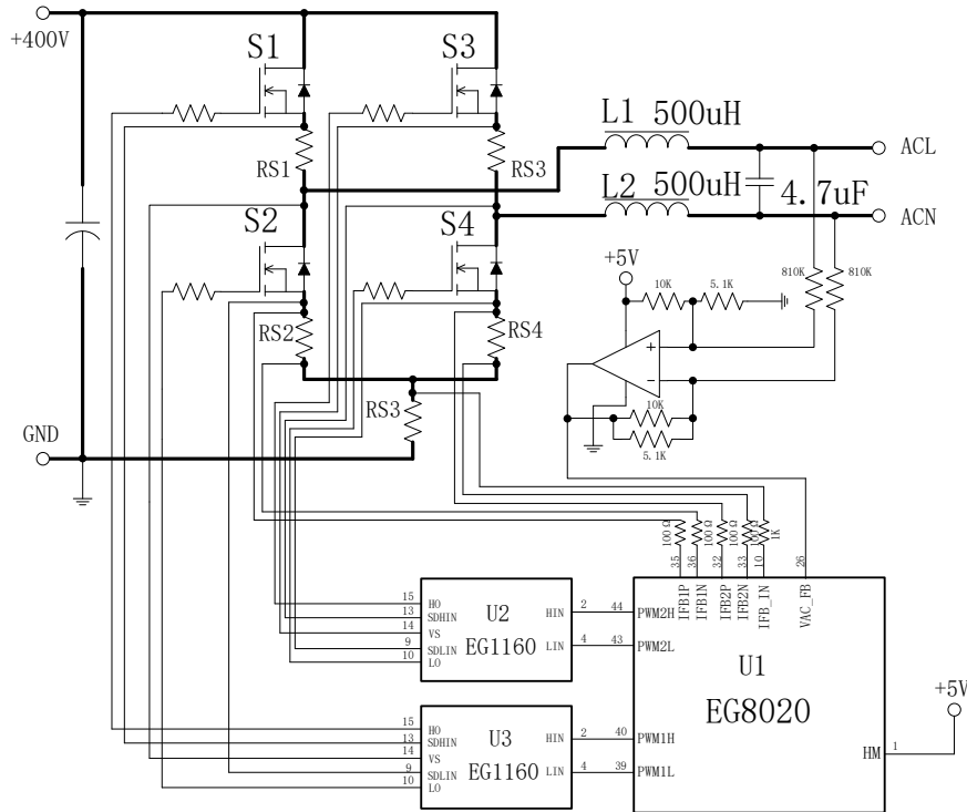
图 8.7b EG8020 的 1 脚输入为“1”时的接线图
