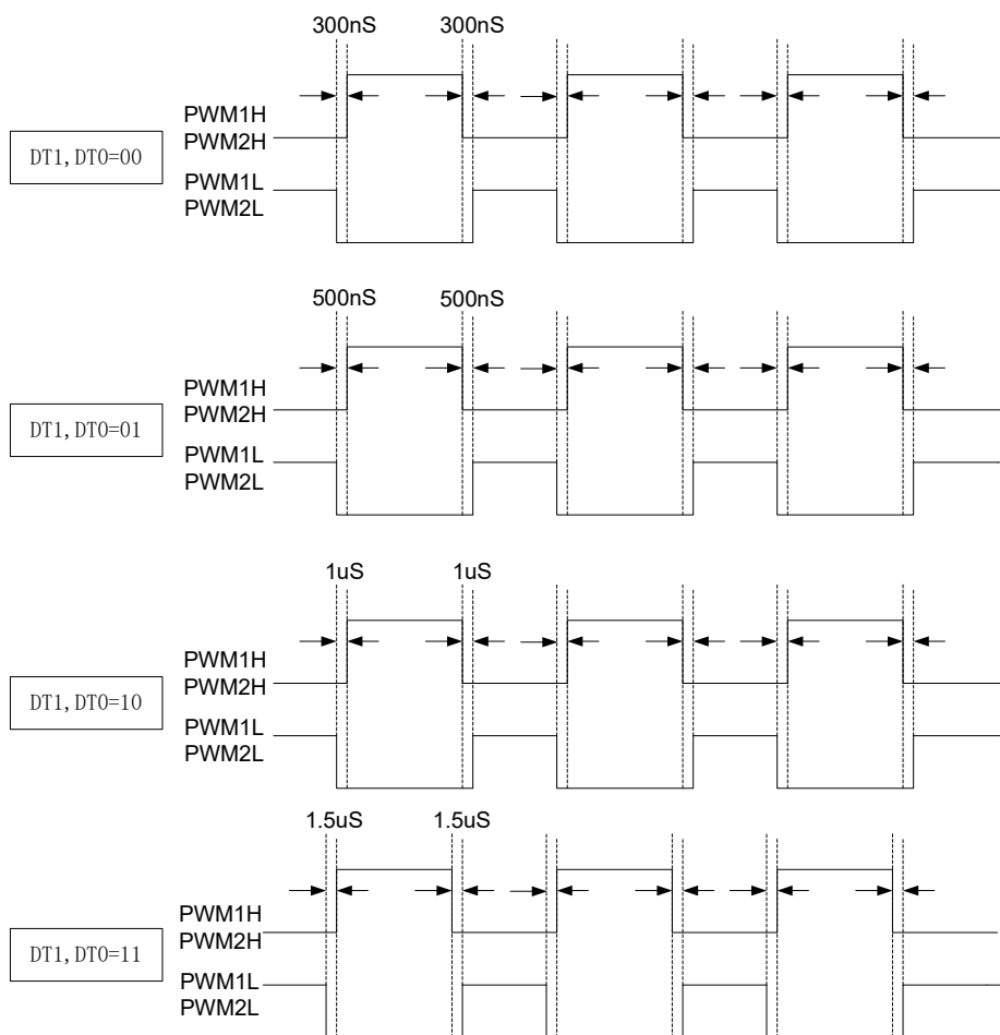
图 8.6a PWM1H、PWM1L 和 PWM2H、PWM2L 死区时间
