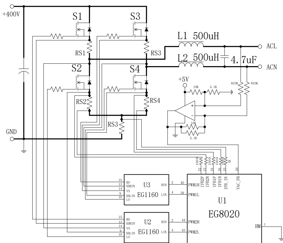
图 8.7a EG8020 的 1 脚输入为“0”时的接线图
