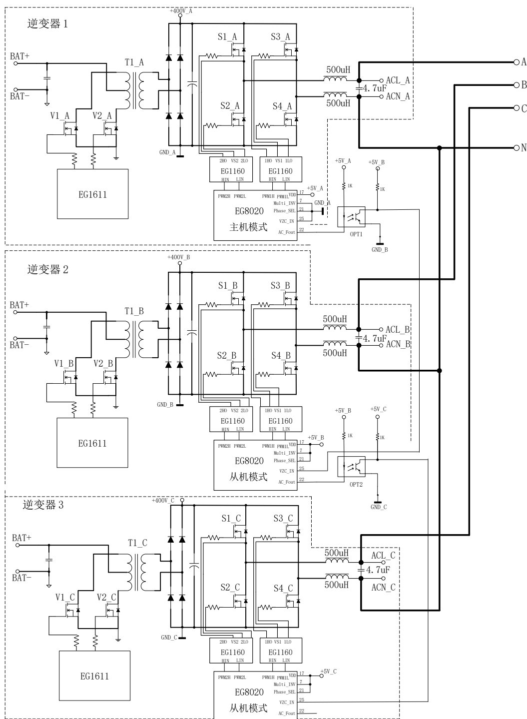
图 10-b. 组三相四线逆变器示意图
