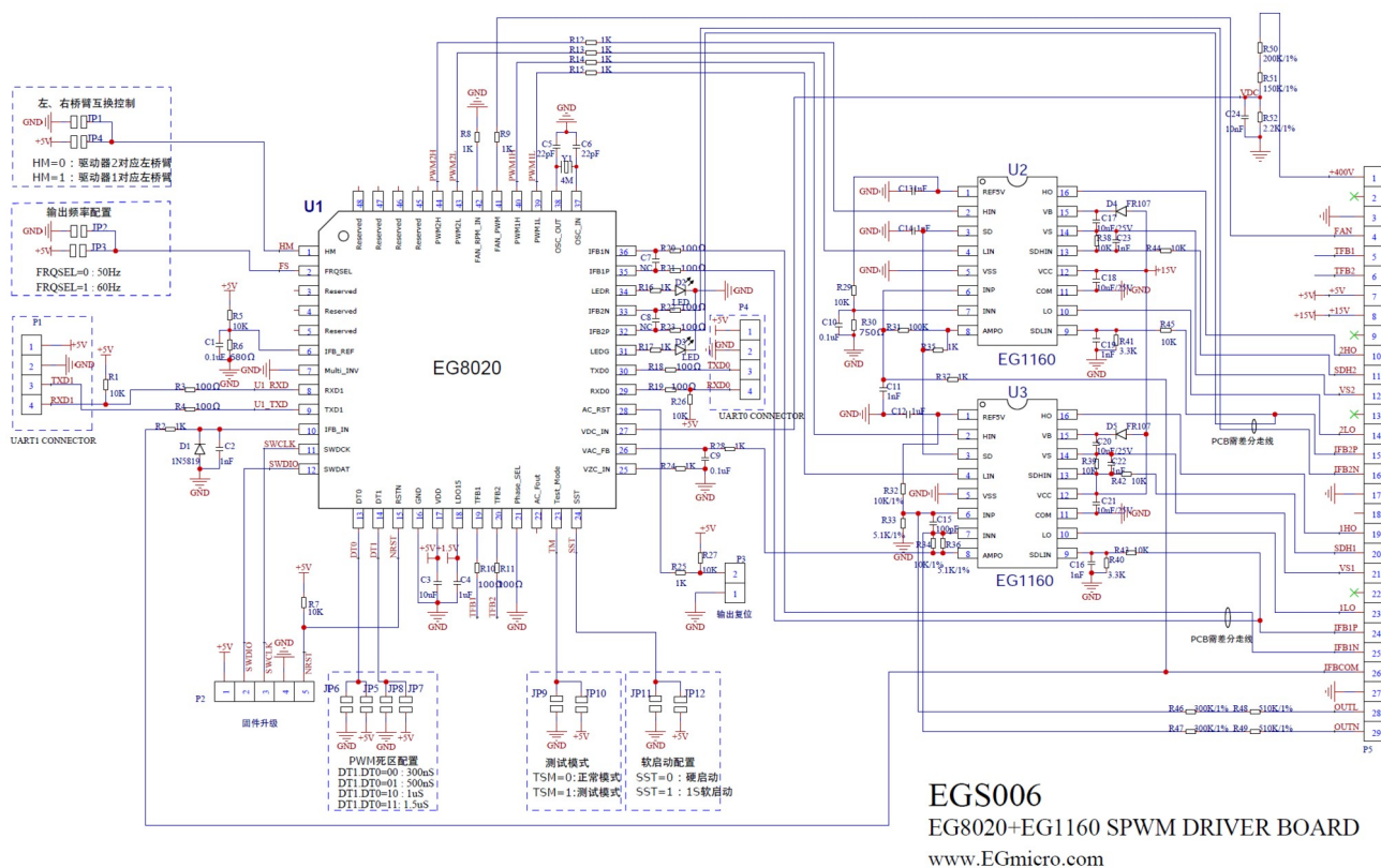
图 6-6. EG8020 后级驱动板原理图
