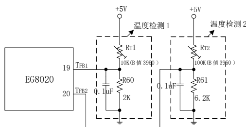
图 8.4a EG8020 的温度检测电路
