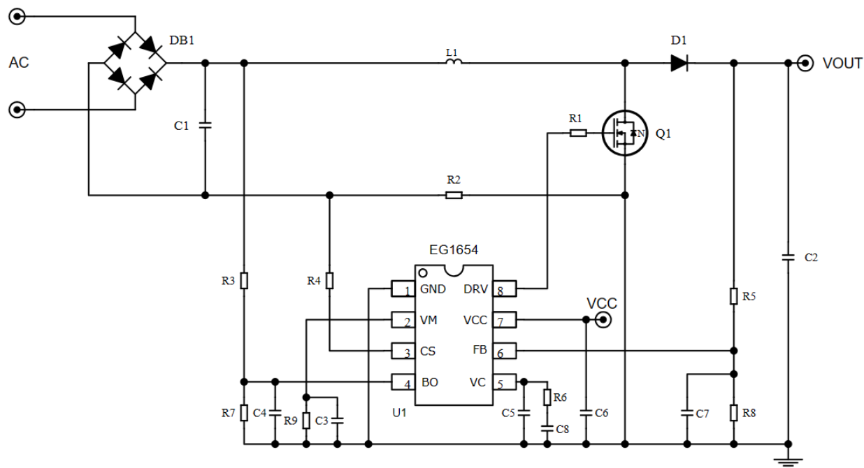
图 6-1. EG1654 有源功率因素校准典型应用图
