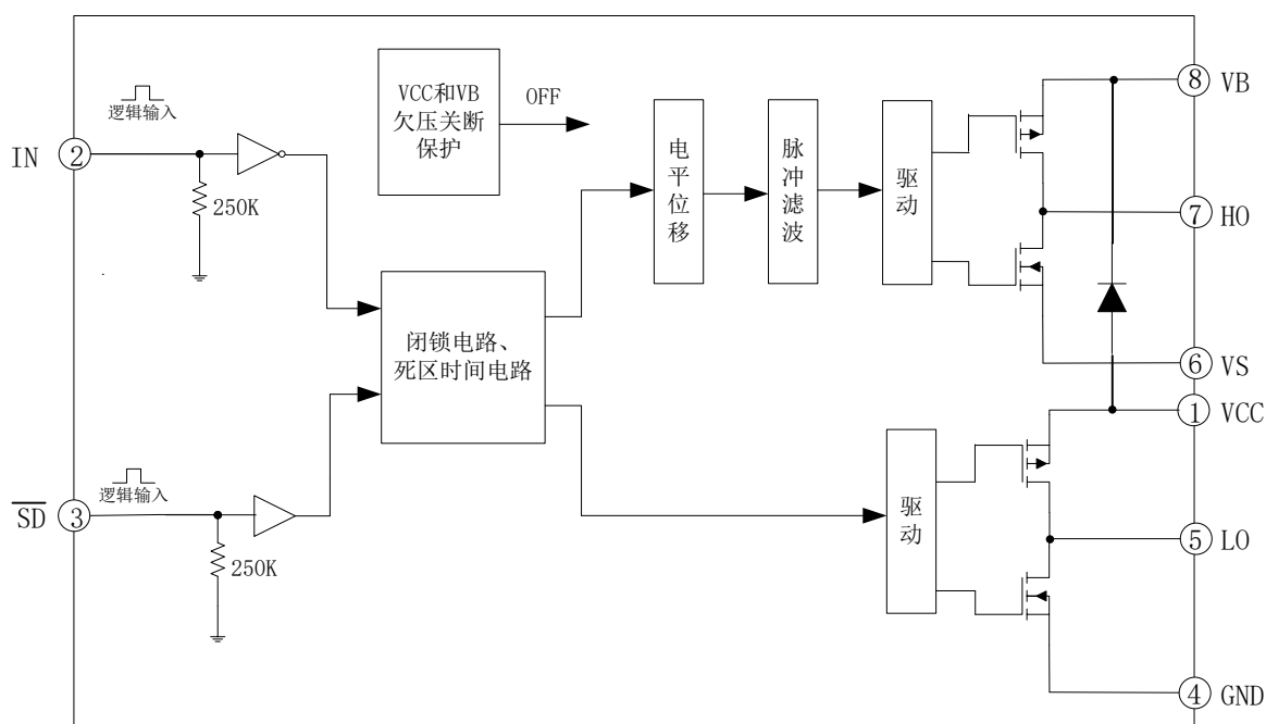
图 5-1. EG2004 内部电路图
