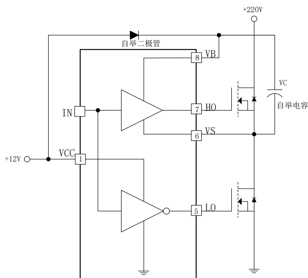
图 8-3. EG2004 自举电路结构
