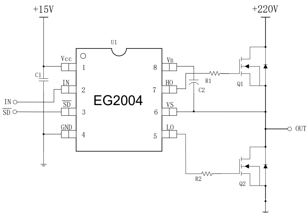
图 6-1. EG2004 典型应用电路图
