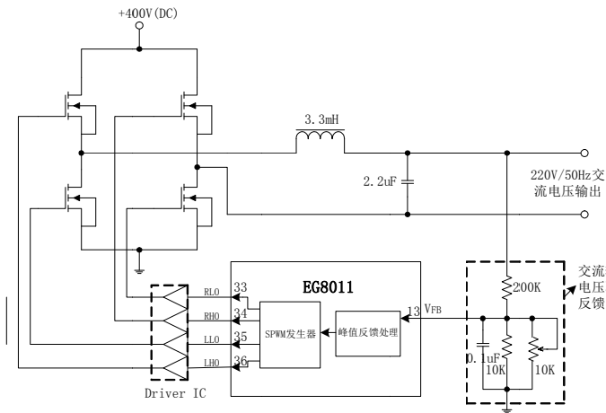
图 7-9a EG8011 单极性调制输出电压反馈电路
